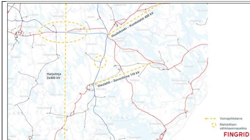
Kuva 1. Maakuntakaavassa esitettävät uudet voimajohtoyhteydet ja sähköasemat
